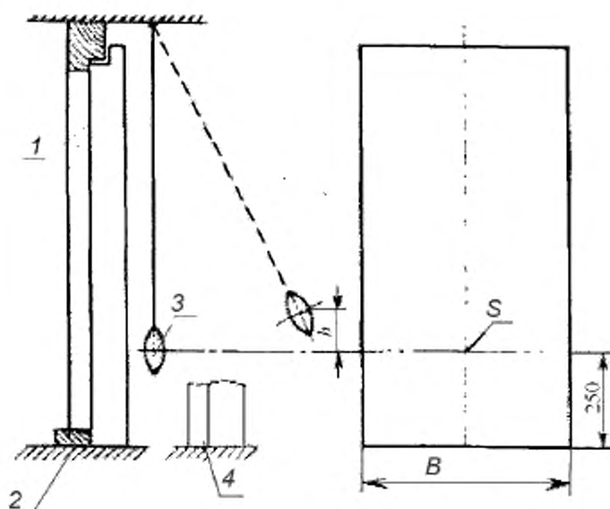
S – центр удара груза; h – высота падения груза; B – ширина двери; 1 – дверное полотно; 2 – коробка с порогом; 3 – неупругое мягкое тело (груз) массой 30 кг; 4 – коробка без порога
