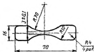
Рисунок 2 — Образец-лопатка типа 2
