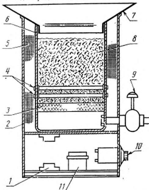
1 — блоки электропроводки и соединителей; 2 — внешний корпус; 3 — пористая пластина; 4 — нагреватель; 5 — изоляция; 6 — внутренний корпус; 7 — фланец; 8 — среда бани; 9 — входной клапан и отверстия для воздуха; 10 — регулятор энергии; 11 — блок надежности
