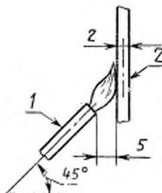
Образец расположен вертикально, пламя контактирует с поверхностью образца
