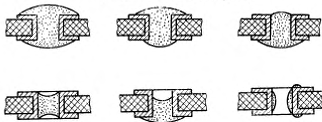
Хорошая паяемость отверстий
