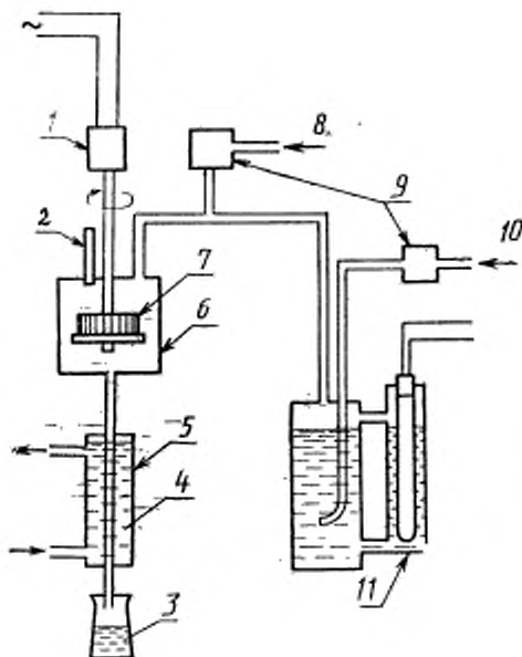
1 — двигатель мешалки; 2 — термометр; 3 — дистиллят; 4 — охлажденная вода; 5 — конденсатор; 6 — камера испытаний; 7 — образцы; 8 — дозируемый газ; 9 — регулятор расходомера; 10 — азот продувной; 11 — па- рогенератор
