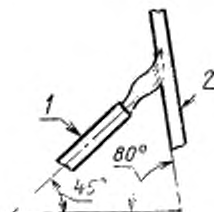
Образец расположен под углом, пламя контактирует с поверхностью образца
