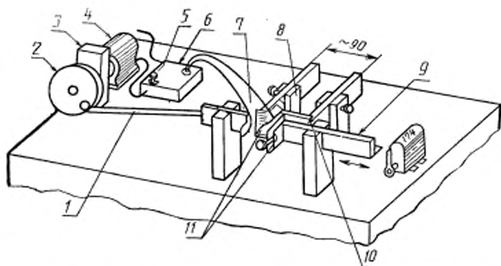
1 — приводной рычаг; 2 — хвостик; 3 — редуктор; 4 — мотор; 5 — установка на нуль; 6 — реле; 7 — испытываемый образец; 8 — непроводящий фиксированный стержень; 9 — непроводящий стержень возвратно-поступательного движения (ход — 75 мм); 10 — петля; 11 — изолированные зажимы
