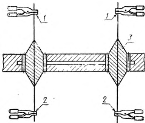
1 — зажимы для измерения тока; 2 — зажимы для измерения напряжения; 3 — вывод
