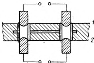
1 — контактные штыри для измерения тока; 2 — контактные штыри для измерения напряжения
