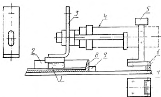
1 — фетровая подложка; 2 — испытуемый образец; 3 — нержавеющая сталь; 4 — поршневой пневматический двигатель; 5 — счетчик; 6 — нержавеющая сталь; 7 — фанера (покрыта лаком); 8 — полдон; 9 — стопор
