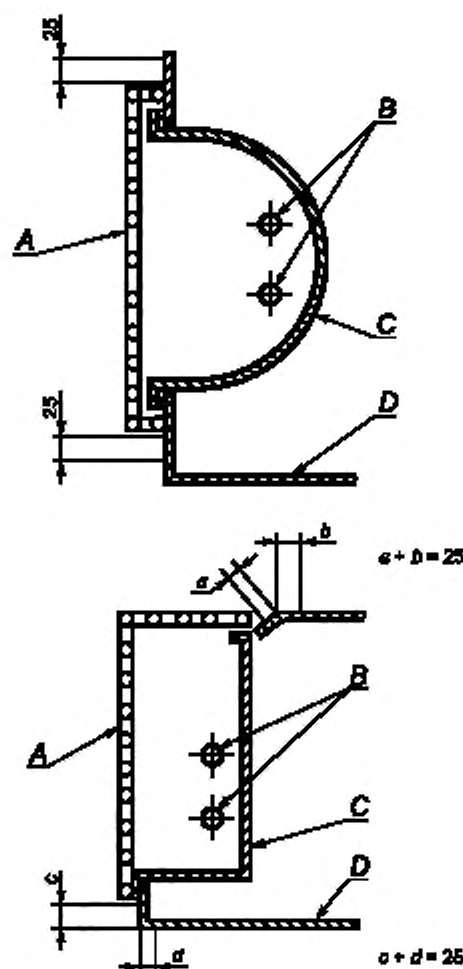
Рисунок 102 — Примеры непосредственного окружения каминных решеток
