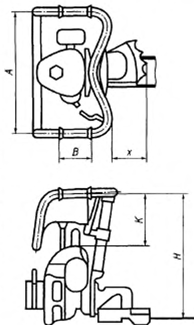
Рисунок 5 — Размеры высокорасположенных рукояток
