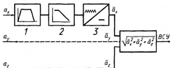
Рисунок В.1 — Взвешенное суммарное ускорение
