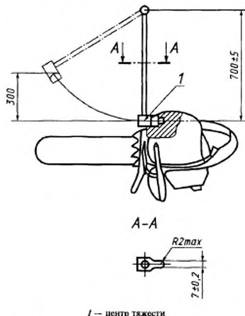
Рисунок А.1 — Маятниковый молоток
