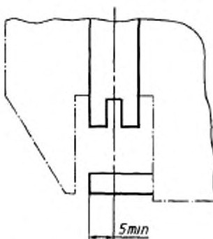
Рисунок 6 — Расположение цепуловителя
