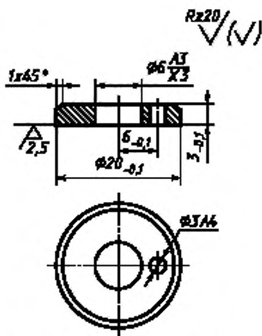
Рисунок Б.3 — Шайба
