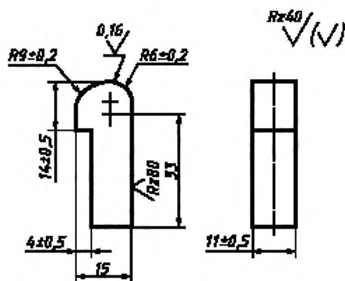
Рисунок А.2 — Губка неподвижная
