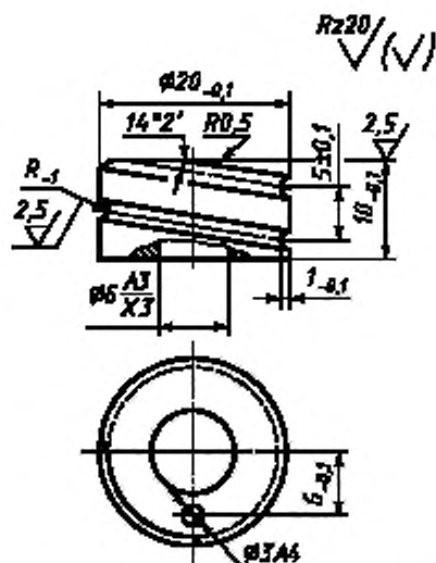
Рисунок Б.2 — «Улитка»
