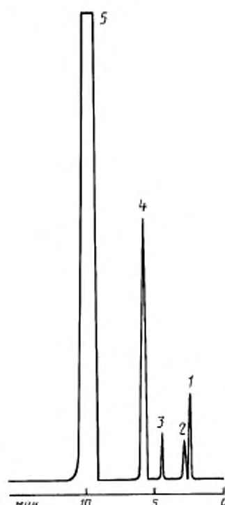
1 — гелий; 2 — водород; 3 — кислород; 4 — азот; 5 — метан
