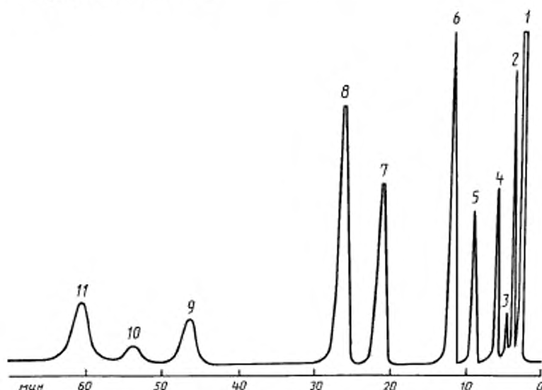
1 — метан+углеводородные газы; 2 — этан; 3 — диоксид углерода; 4 — пропан; 5 — n -бутан; 6 — n -бутан; 7 — n -пентан; 8 — n -пентан; 9 — 2-метилпентан+2,3-диметилбутан; 10 — 3-метилпентан; 11 — n -гексан
