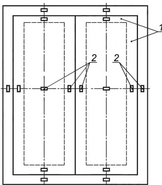
1 — однородные зоны; 2 — тепломеры и термодпары Рисунок 3 — Рекомендуемое расположение датчиков при испытании дверного блока
