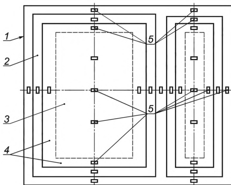
1 — рама; 2 — створка; 3 — стеклопакет; 4 — однородные зоны; 5 — тепломеры и термодпары Рисунок 2 — Рекомендуемое расположение датчиков при испытании оконного блока
