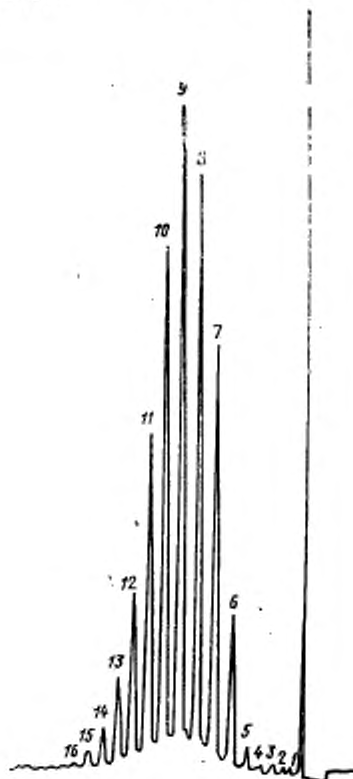
Обозначения пиков спиртов:
