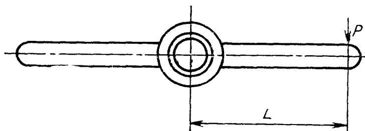
Схема измерения момента вращения
