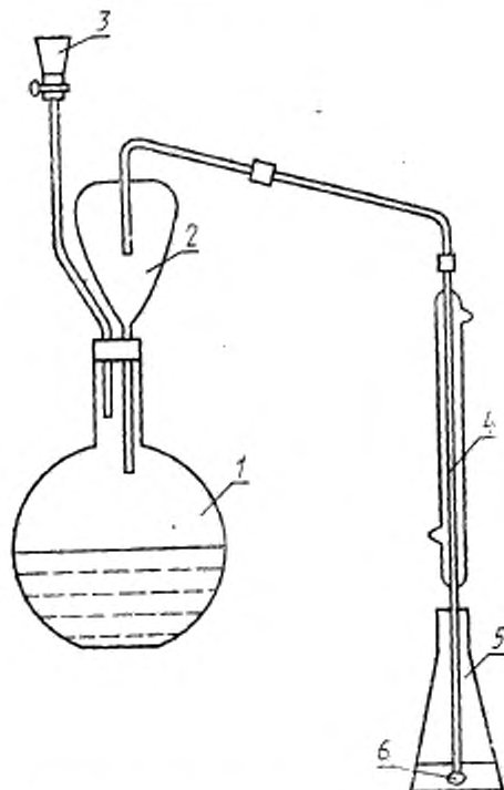
1 — реакционная колба вместимостью 250—300 см 3 ; 2 — каплеуловитель; 3 — капельная воронка с краном; 4 — холодильник; 5 — приемник; 6 — барботер
