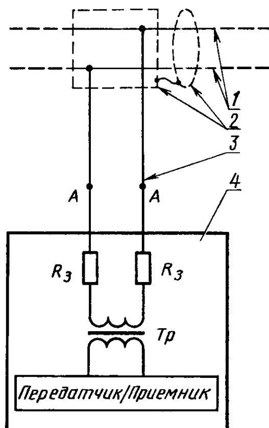
Электрическая схема подключения ответвителя без согласующего трансформатора к магистральной шине
