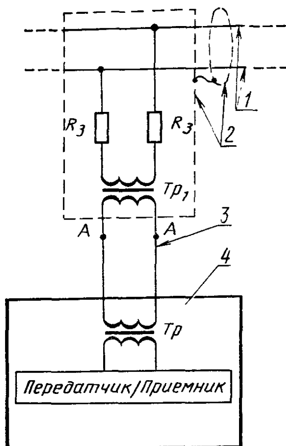
Электрическая схема подключения ответвителя с согласующим трансформатором к магистральной шине
