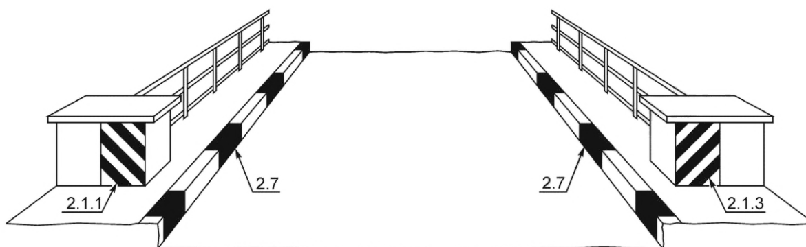
Рисунок В.23 — Пример нанесения разметки 2.1.1, 2.1.3 и 2.7
