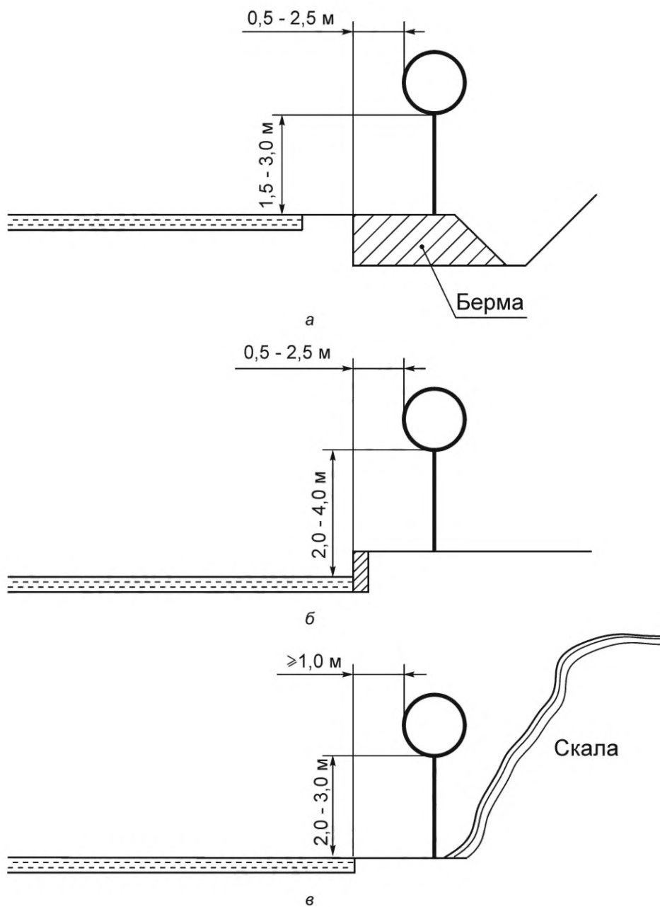
Рисунок В.1 — Типовое размещение знаков в поперечном профиле дороги
