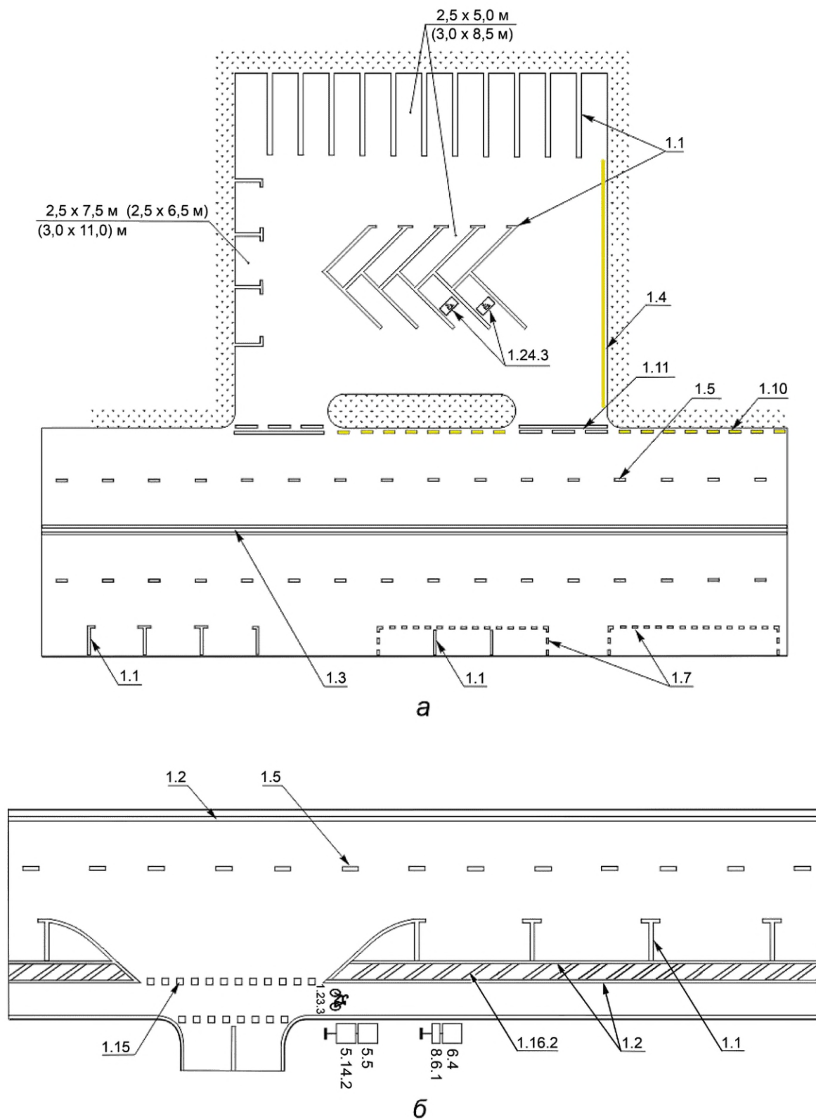
a — пример нанесения разметки в местах организованной парковки транспортных средств на проезжей части и прилегающей территории; б — пример нанесения разметки в местах организованной парковки транспортных средств с устройством велополосы
