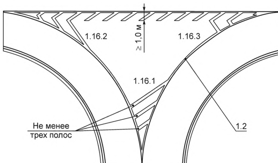
Рисунок В.12 — Пример нанесения разметки 1.16.1—1.16.3
