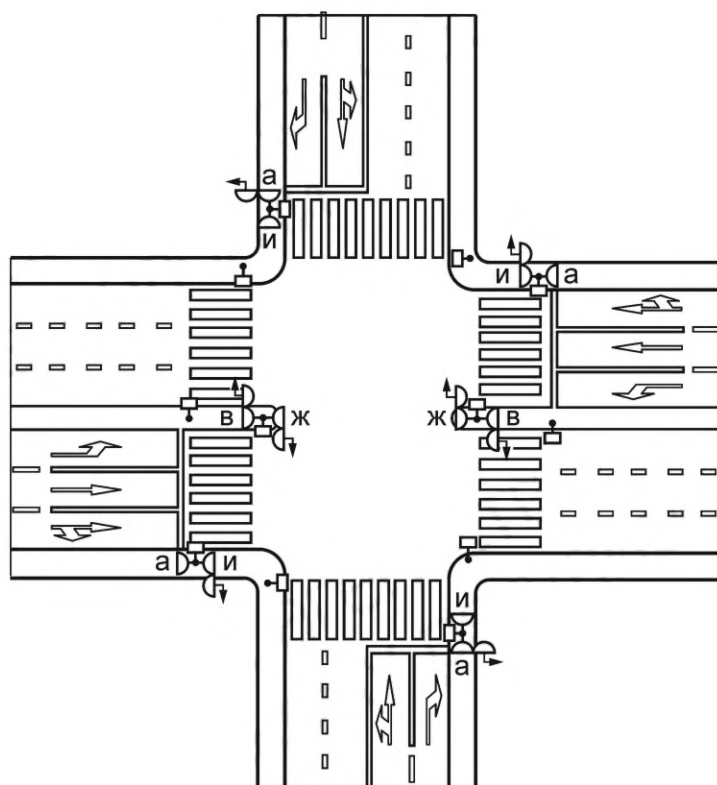
Рисунок В.26 — Места установки светофоров
