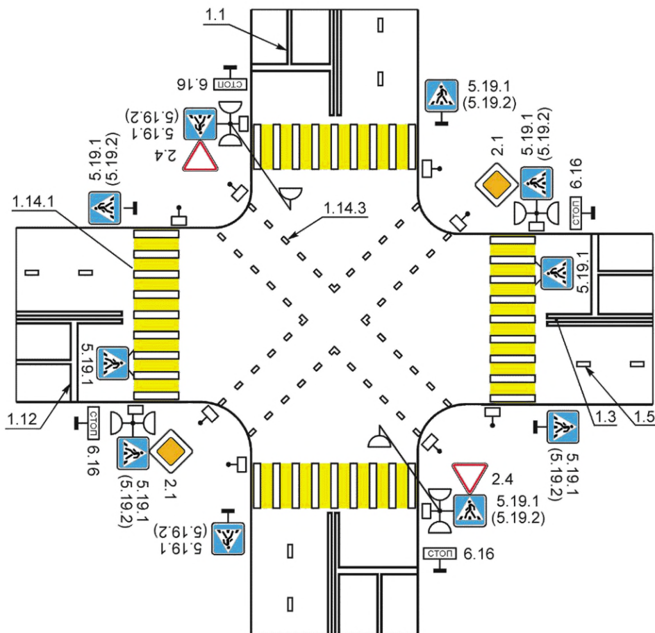
Рисунок В.19 — Пример нанесения диагонального пешеходного перехода
