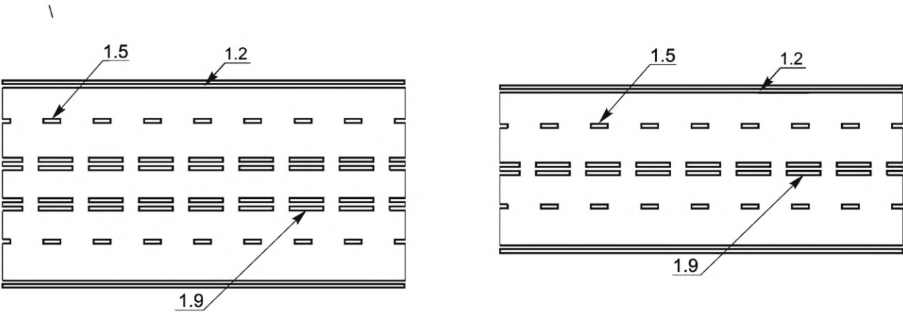
Рисунок В.17 — Примеры нанесения разметки 1.9
