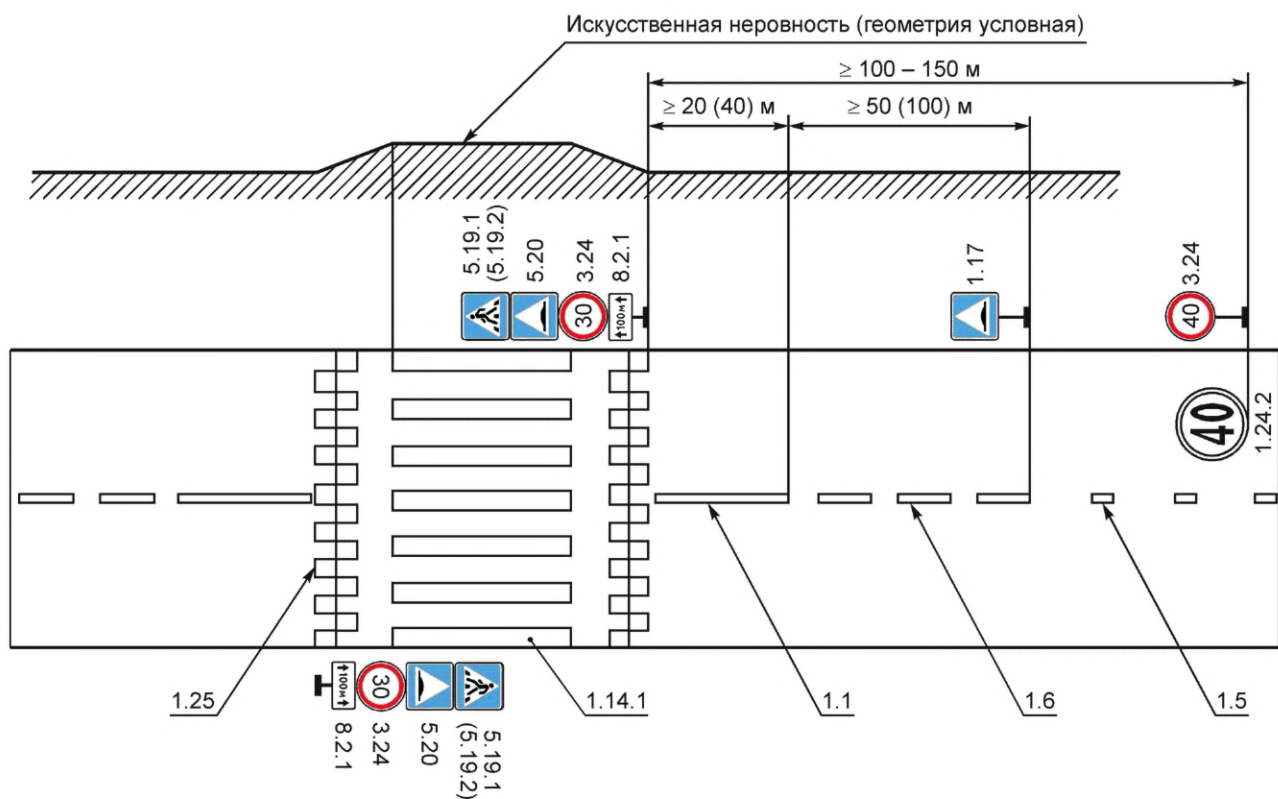
Рисунок В.21 — Пример нанесения разметки 1.25
