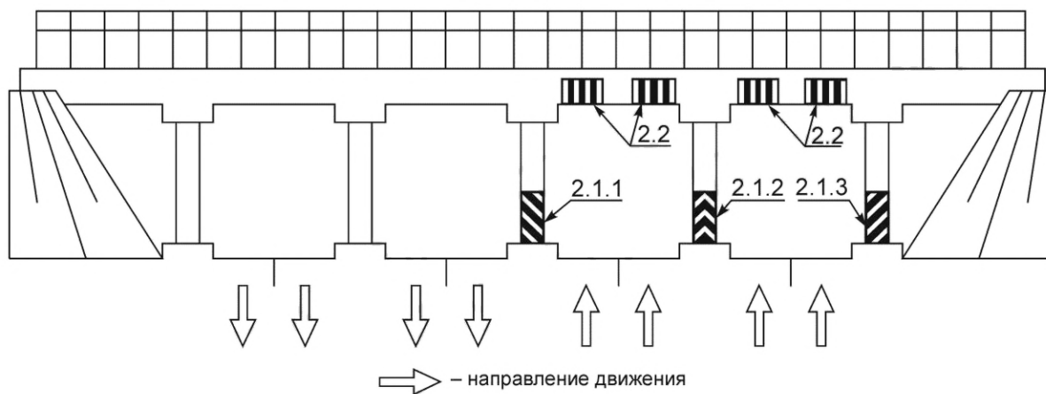
Рисунок В.22 — Пример нанесения разметки 2.1 и 2.2
