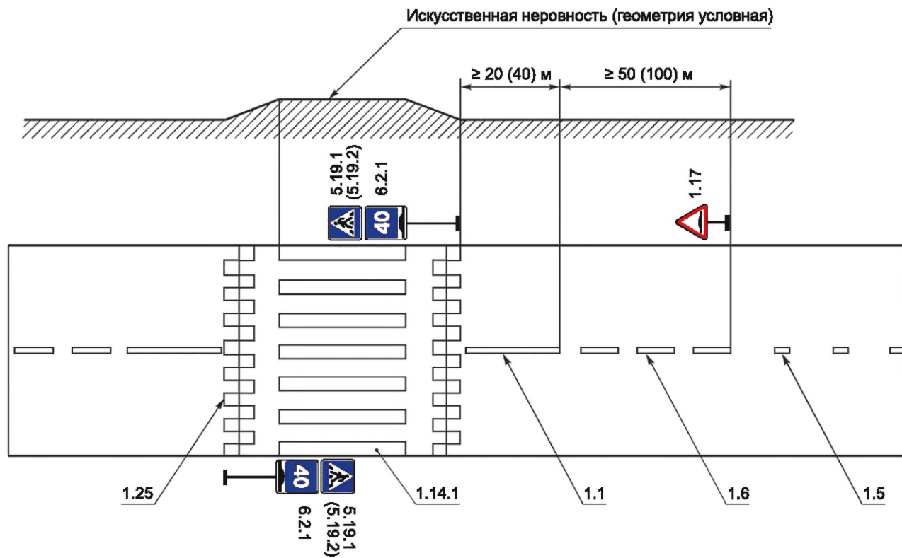
Рисунок В.21 — Примеры нанесения разметки 1.25».
