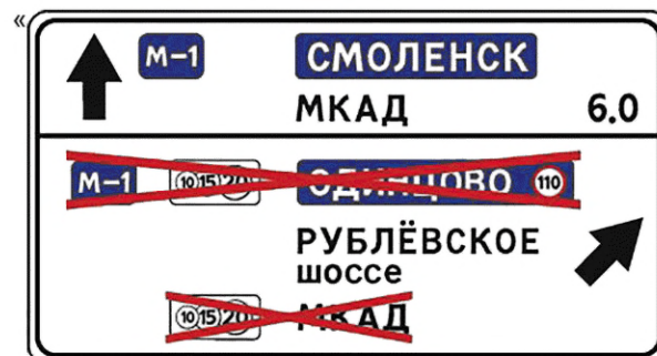
В.31 — Пример зачехления надписей способом перечеркивания».
