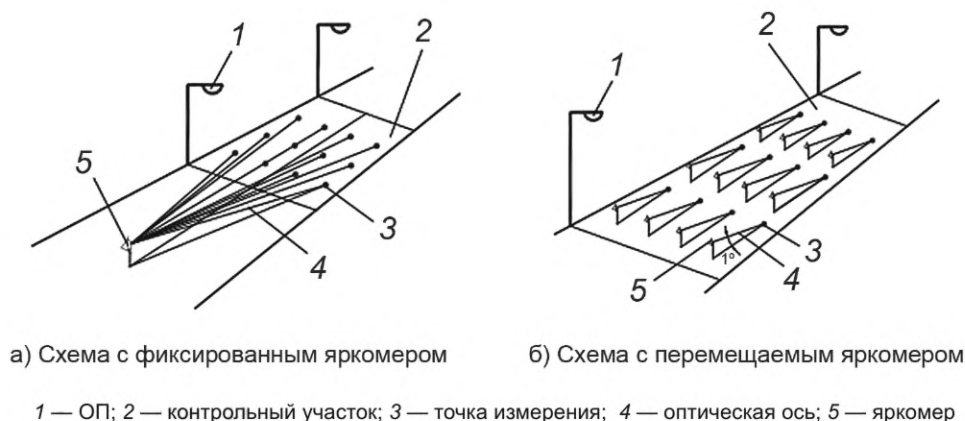
Рисунок 1 — Расположение контрольного участка при измерении средней яркости дорожного покрытия
