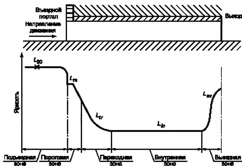
Рисунок Б.4 — Схема расположения яркостных зон в туннеле ( L_{\lambda_0} , L_{th} , L_{tr} , L_{im} , L_{ax} — по [1])
