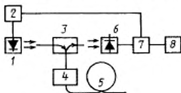
1—источник излучения; 2—генератор электрических импульсов; 3—направленный ответвитель; 4—устройство ввода; 5—измеряемый кабель; 6—приемник излучения; 7—устройство обработки сигнала; 8—регистрирующая система
