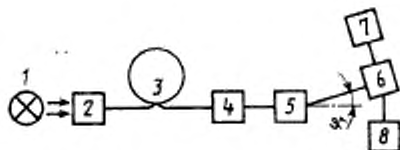
1—источник излучения; 2—устройство ввода; 3—измеряемый кабель; 4—фильтр мод оболочки; 5—устройство крепления; 6—приемник излучения; 7—устройство перемещения; 8—регистрирующее устройство
