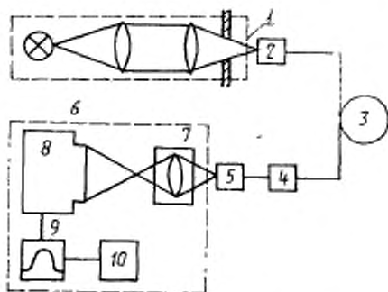
1—источник излучения; 2—устройство ввода; 3—измеряемый кабель; 4—фильтр мод оболочки; 5—устройство крепления; 6—регистрирующее устройство; 7—микроскоп; 8—телевизионная камера; 9—монитор; 10—блок управления
