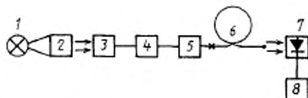
1—источник излучения (лампа накаливания); 2—монокроматор; 3—устройство ввода; 4—смеситель мод; 5—фильтр мод оболочки; 6—оптический кабель; 7—приемник излучения; 8—регистрирующее устройство
