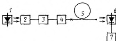
1—источник излучения; 2—устройство ввода; 3—смеситель мод; 4—фильтр мод оболочки; 5—оптический кабель; 6—приемник излучения; 7—регистрирующее устройство
