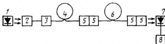
1—источник излучения; 2—устройство ввода; 3—смеситель мод; 4—вспомогательное оптическое волокно; 5—оптические разъёмные соединители; 6—измеряемый кабель; 7—приёмник излучения; 8—регистрирующее устройство
