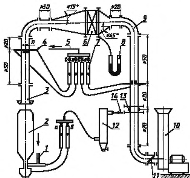
1 — дозатор пыли; 2 — классификатор—генератор аэрозолей; 3 — входной коллектор; 4 — пылезборные трубки; 5 — вакуумный насос; 6 — испытываемый воздухоочиститель; 7 (н, г, д, е) — ротаметры; 8 — микроманометр; 9 — трубопровод; 10 — вентилятор стенда; 11 — дроссель-клапан; 12 — электрофильтр; 13 — диафрагма; 14 — нагревательный трубопровод
