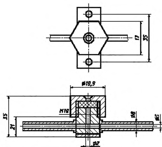
Рисунок А.6 — Пробоотборник
