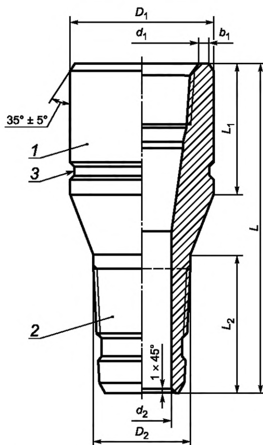
1 — муфтовый конец; 2 — ниппельный конец; 3 — маркировочный пояс
