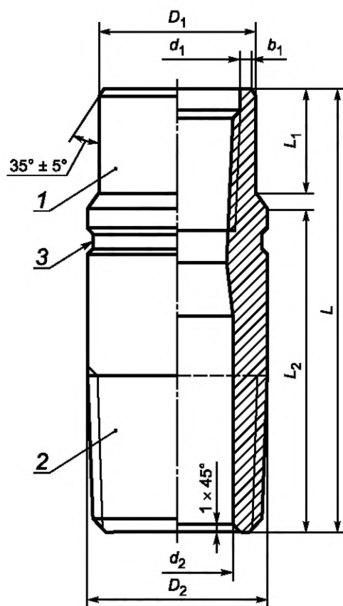
1 — муфтовый конец; 2 — ниппельный конец; 3 — маркировочный пояс
