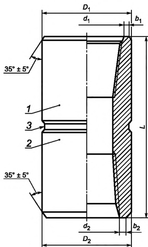
1 — верхний конец; 2 — нижний конец; 3 — маркировочный пояс
