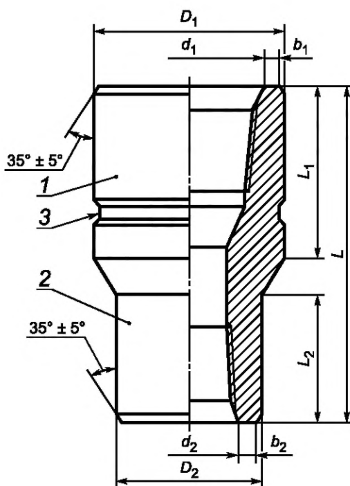
1 — верхний конец; 2 — нижний конец; 3 — маркировочный пояс
