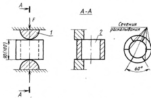
1—колец; 2—образец
