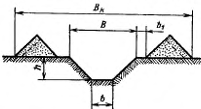
h —глубина канала; b —ширина канала по дну; B —ширина канала по верху; B_k —ширина основания кавальера (ширина разбрасывания); b_1 —ширина бермы
