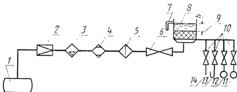
1—источник сжатого воздуха; 2—редукционный клапан; 3—влаго-маслоотделитель; 4—осушитель; 5—фильтр; 6—кран точной регулировки; 7—сливная трубка для установки уровня жидкости над образцом; 8—испытуемый образец; 9—держатель для крепления образцов; 10—кран; 11—манометр Мо 0,4 МПа по ГОСТ 6521—72; 12—манометр Мо 0,16 МПа по ГОСТ 6521—72; 13—U-образный манометр, заполненный водой; 14—микроманометр ММН-2400(5)—0,6 ГОСТ 11161—84.
