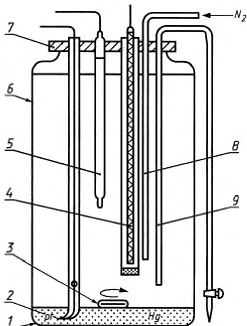
1 — рабочий ртутный электрод; 2 — платиновый контакт; 3 — магнитная мешалка; 4 — вспомогательный электрод из спектрального угля; 5 — хлорсеребряный электрод сравнения; 6 — полистирольный сосуд; 7 — крышка; 8 — стеклянная трубка для подвода азота; 9 — сифон для слива электролита
