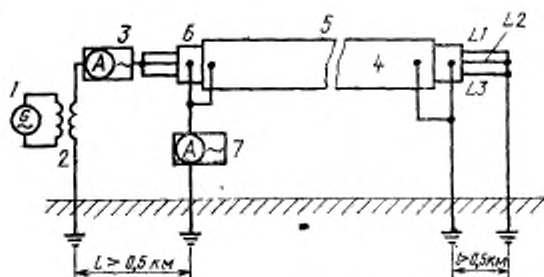
1 — генератор; 2 — согласующий трансформатор; 3 — устройство для измерения величины тока в жилах кабеля; 4 — силовоточный кабель; 5 — броня; 6 — оболочка; 7 — устройство для измерения величины тока в оболочке и в броне; L 1 , L 2 , L 3 — жила сильноточного кабеля; L — расстояние между устройствами заземления
