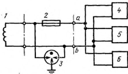
1 — трансформатор; 2 — предохранитель; 3 — трехфазный разрядник защиты от перенапряжений; 4 — селективный вольтметр (анализатор гармоник); 5 — вольтметр для измерения эффективных значений; 6 — психофотометр
