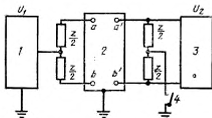
1 — генератор с очень малым внутренним сопротивлением; 2 — измеряемый объект; 3 — вольтметр; 4 — выключатель для регистрации продольной несимметрии; Z — волновое сопротивление измеряемого объекта
