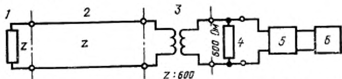
1 — сторона, противоположная месту измерения; 2 — линия связи с волновым сопротивлением Z ; 3 — согласующий трансформатор; 4 — сопротивление нагрузки 600 Ом; 5 — псофометр; 6 — самоизлучающий измерительный прибор
