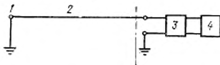
1 — конец, противоположный месту измерения; 2 — линия связи или измерительная цепь; 3 — вольтметр; 4 — самопишущий измерительный прибор Черт. 7
