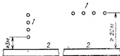
1 — стержни заземления; 2 — металлическое сооружение, проложенное в земле
