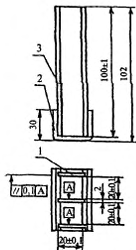
Рисунок 5 — Форма размером 20x20x100 мм
