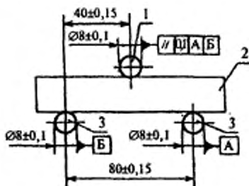
Рисунок 7 — Схема расположения образца-балочки при испытании
