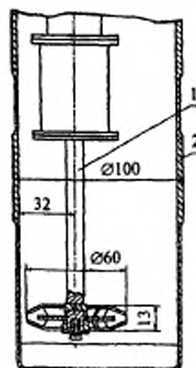
1 - лопастное устройство; 2 - стакан Рисунок 1 - Смеситель лопастной
