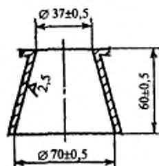
Рисунок 2 — Форма-конус
