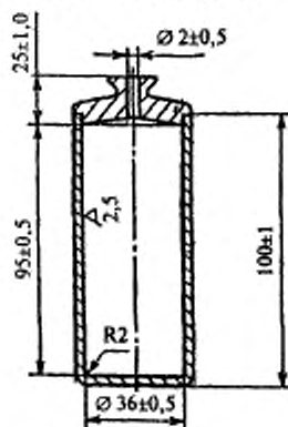
Рисунок 3 — Пикнометр
