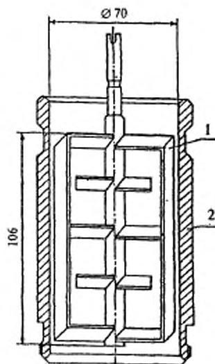
1 — лопастное устройство; 2 — стакан
