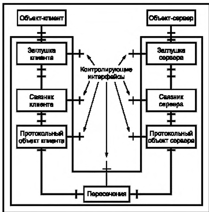
Рисунок 2 — Пример базового канала клиент/сервер
