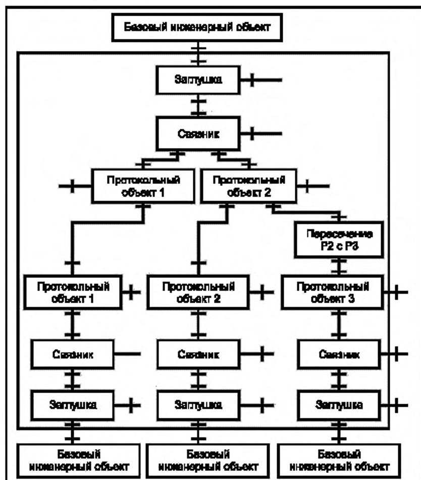
Рисунок 3 — Пример канала с несколькими оконечными точками
