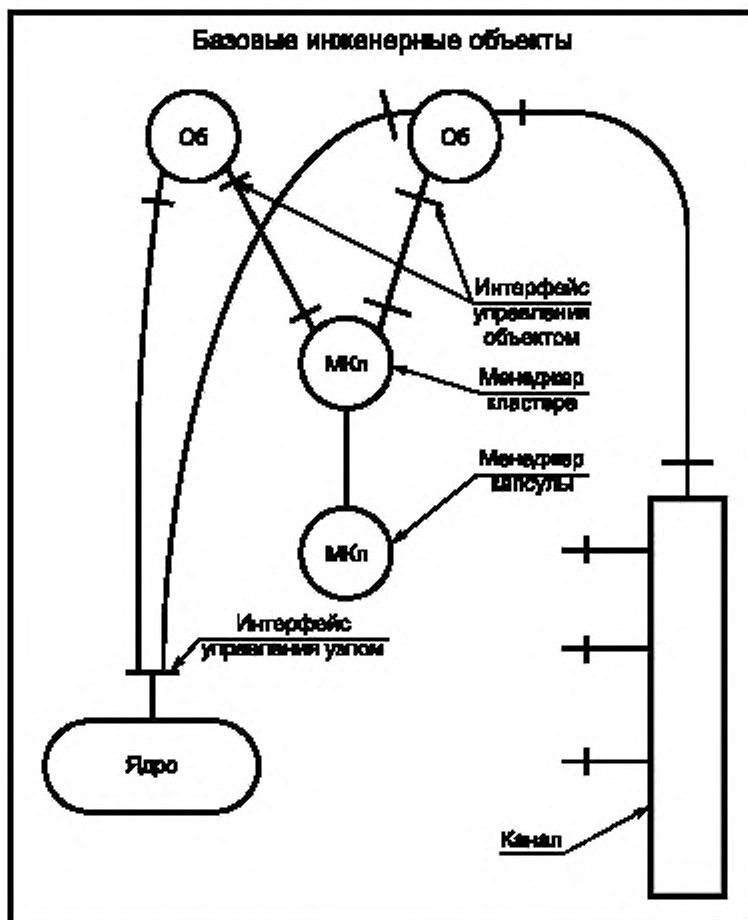
Рисунок 4 — Пример структуры, поддерживающий базовый инженерный объект
