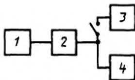
1 — источник электроэнергии переменного (постоянного) тока; 2 — генератор импульсов; 3 — проверяемая аппаратура; 4 — электронный осциллограф
