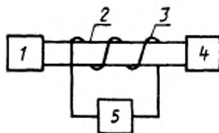
1 — эквивалент источника сигнала по входу и эквивалент нагрузки по выходу; 2 — жгут линий связи; 3 — провод-индуктор; 4 — проверяемая аппаратура; 5 — генератор низкой частоты
