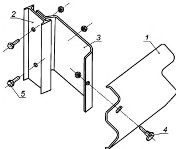
1 — балка; 2 — стойка; 3 — консоль-амортизатор; 4 — болт M16 x 45.5.8; 5 — болт M16 x 30.5.8
