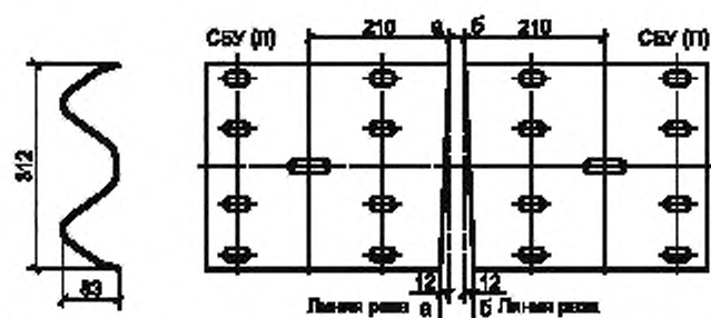
СБУ (П) — правая; СБУ (Л) — левая (зеркальное изображение правой)
