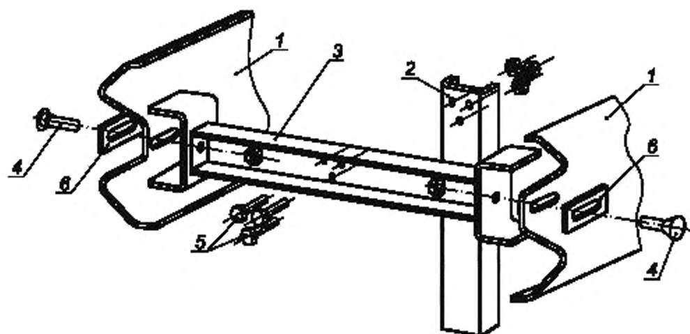
1 — балка; 2 — стойка; 3 — консоль-распорка; 4 — болт М16 × 45.5.8; 5 — болт М16 × 30.5.8; 6 — шайба 80 × 40 × 4 мм
