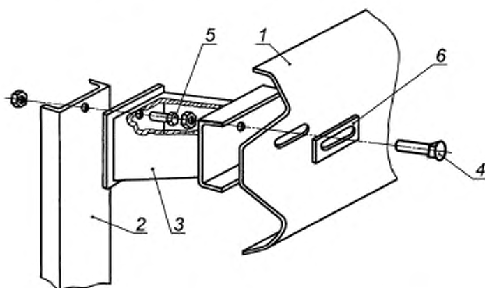
1 — балка; 2 — стойка; 3 — консоль жесткая; 4 — болт М16 × 45.5.8; 5 — болт М16 × 30.5.8; 6 — шайба 80 × 40 × 4 мм
