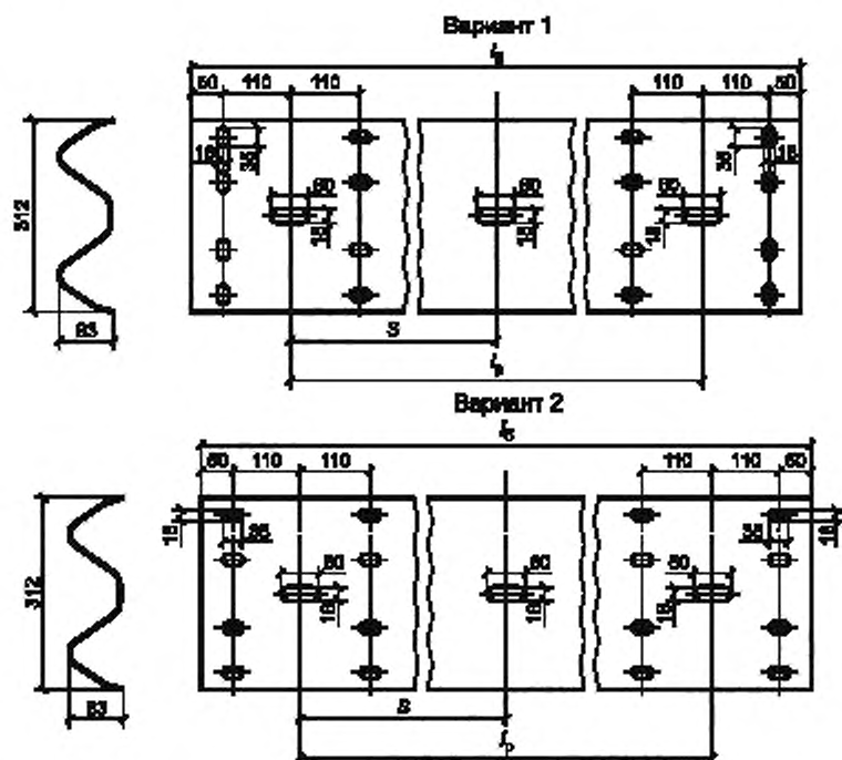
Рисунок 4 — Секция балки ограждений СБ
