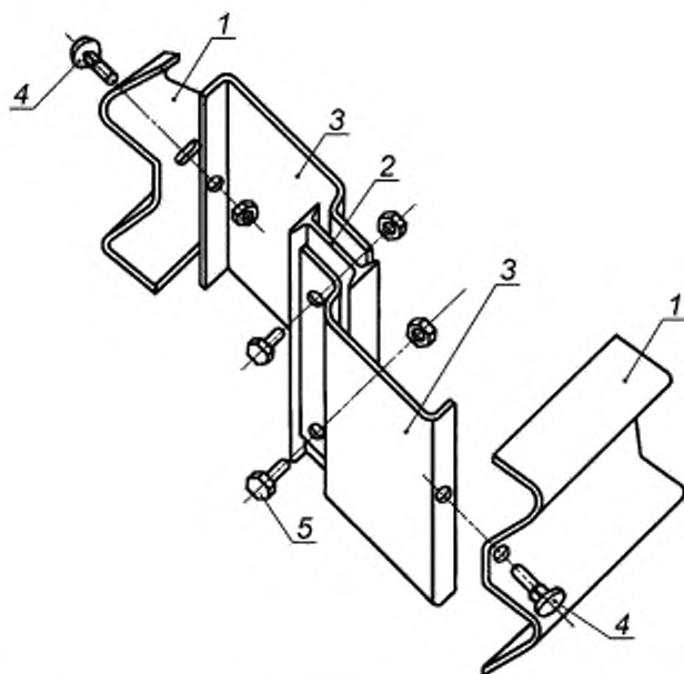
1 — балка; 2 — стойка; 3 — консоль-амортизатор; 4 — болт M16 x 45.5.8; 5 — болт M16 x 30.5.8
