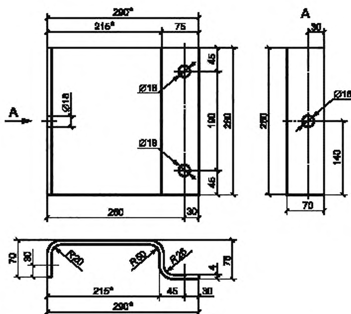
Рисунок 11 — Консоль-амортизатор КА
