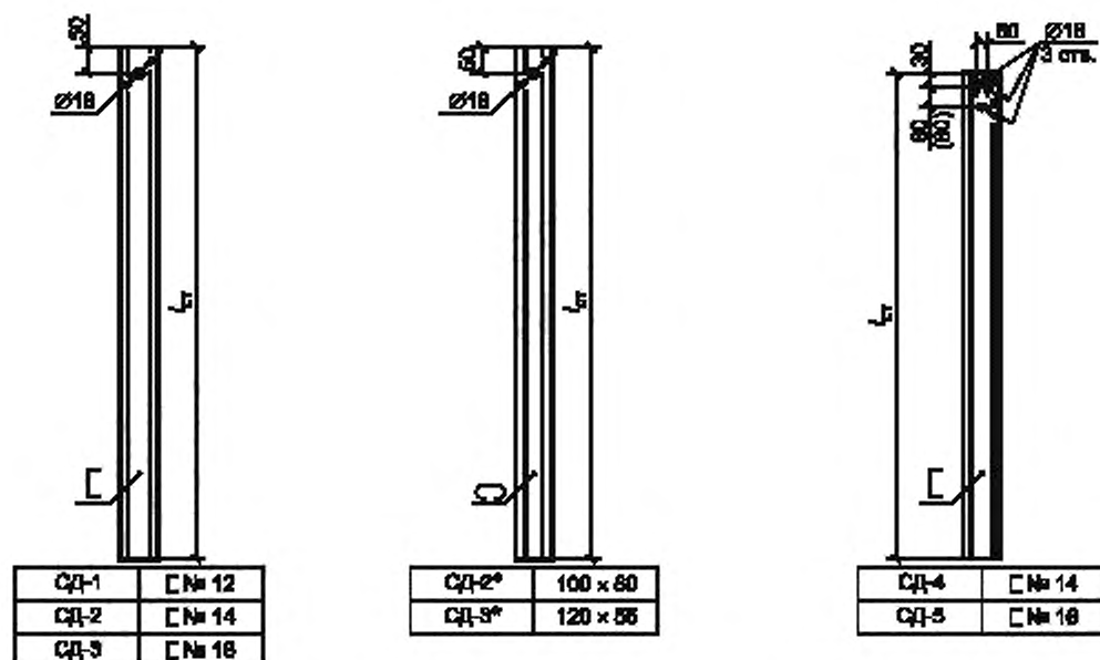
а) Для односторонних ограждений с жесткими консолями
