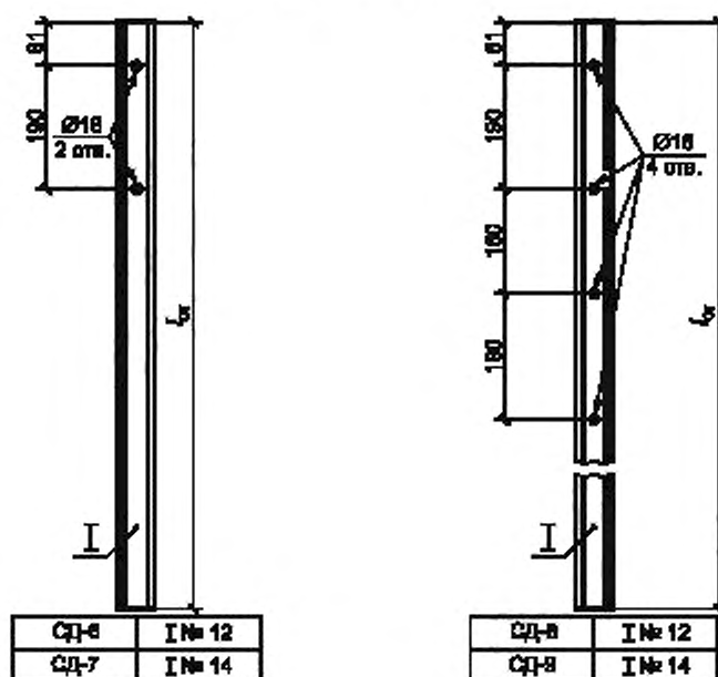
г) Для односторонних ограждений с консольно-амортизатором с одним ярусом балки
