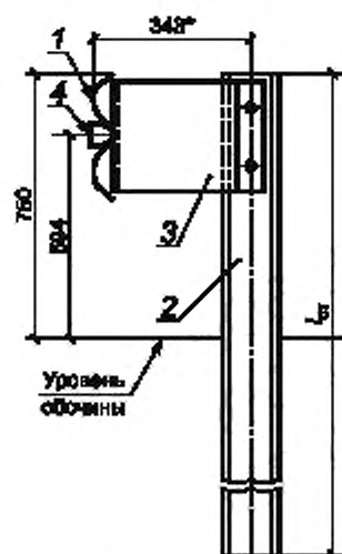
а) Одностороннее одностроное ограждение
