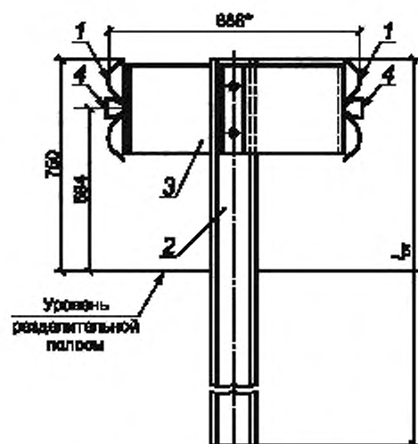
б) Двустороннее одностроное ограждение
