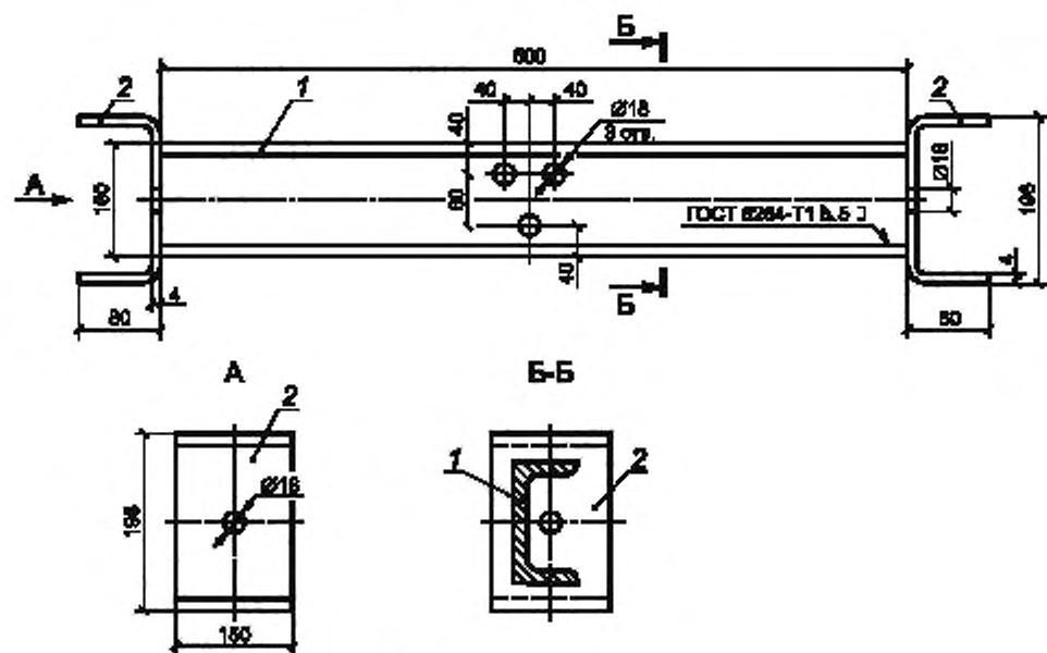
Рисунок 9 — Консоль-распорка КР
