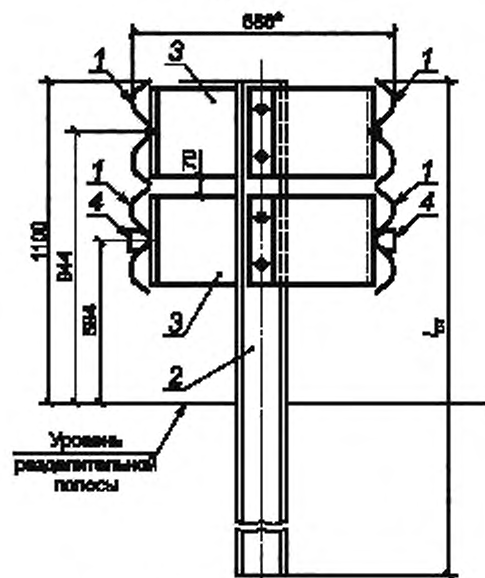
г) Двустороннее двухстороннее ограждение
