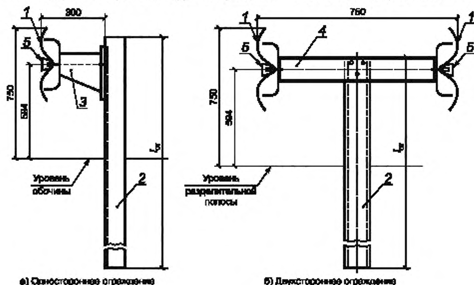
Рисунок 1 — Конструкция ограждений дорожной группы с жесткими консолями
