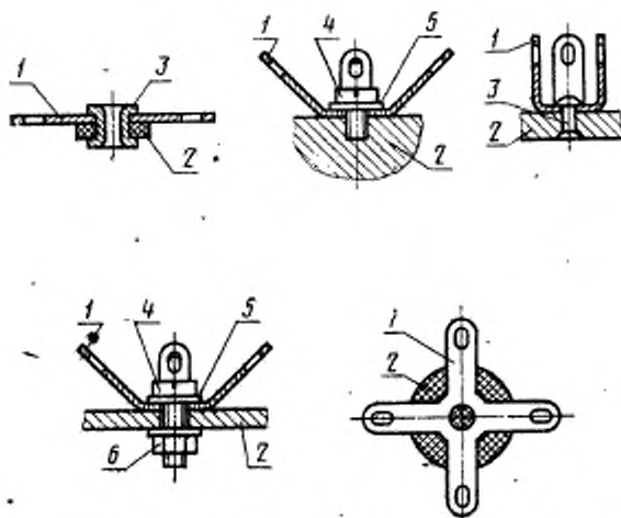
1—лепесток; 2—основание; 3—заклепка; 4—винт; 5—шайба; 6—рейка.
