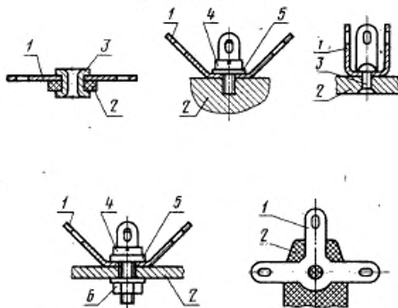
1—лепесток; 2—основание; 3—защелка; 4—винт; 5—шайба; 6—гайка
