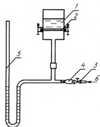
Схема установки для определения класса фильтра
