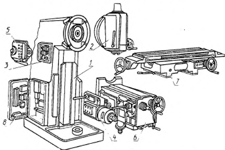
1—станка; 2—поворотная головка; 3—коробка скоростей; 4—коробка подач; 5—коробка переключения; 6—консоль; 7—стол и салазки; 8—электрооборудование.
