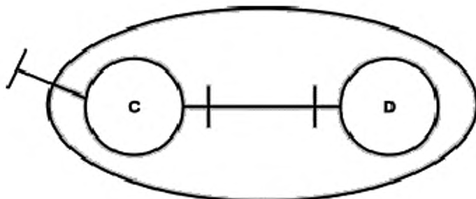
Рисунок 1 — Композиция объектов
