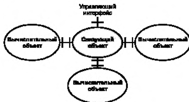
Рисунок 2 — Составное связывание
