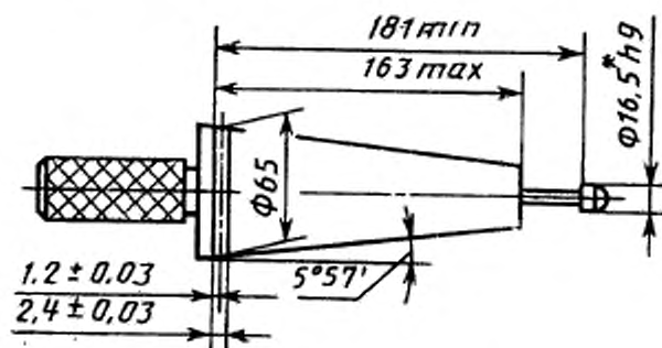
Калибр для патрона с закругленным торцем
