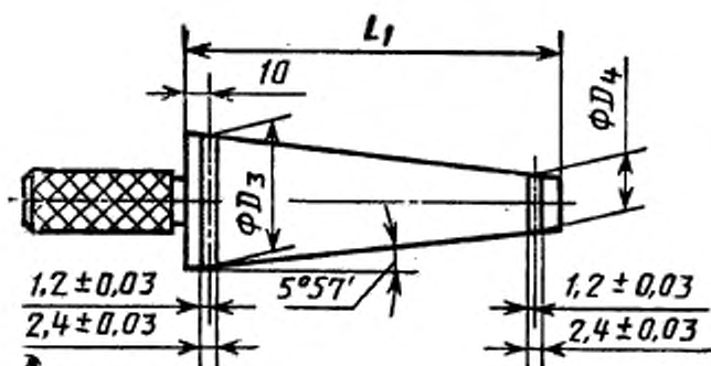
Калибр для патрона с закругленным торцем
