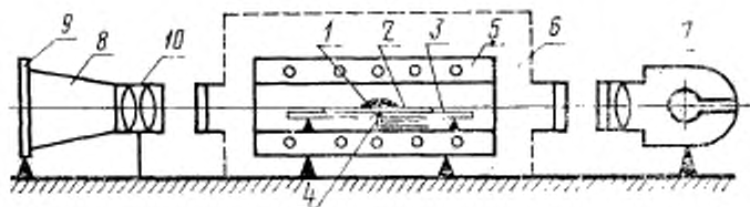
Схема установки для проведения испытаний
