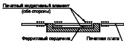
Рисунок Г.6 — Размещение одного из ферритовых сердечников
