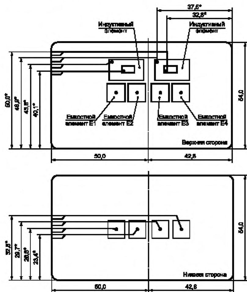
Рисунок Г.1 — Испытательная карта
