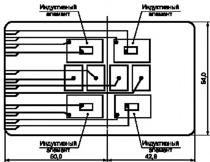
Рисунок Г.4 — Испытательное считывающее устройство
