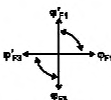
Рисунок 3 — Сдвиг фаз. Вариант 2
