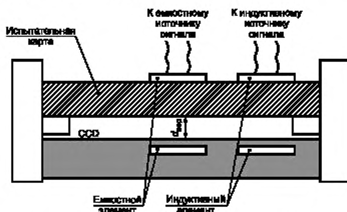
Рисунок Г.10 — Схема установки для испытаний CCD
