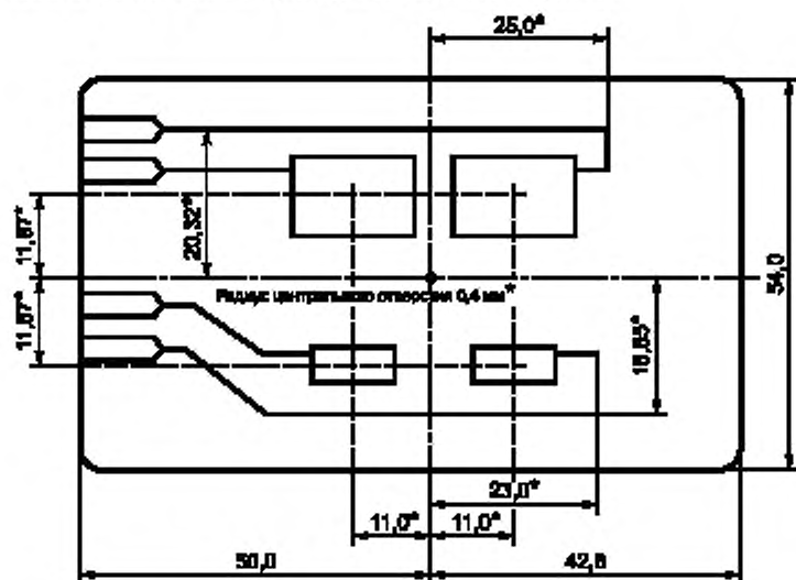
Рисунок Г.3 — Испытательная вставка с малыми измерительными индуктивными элементами
