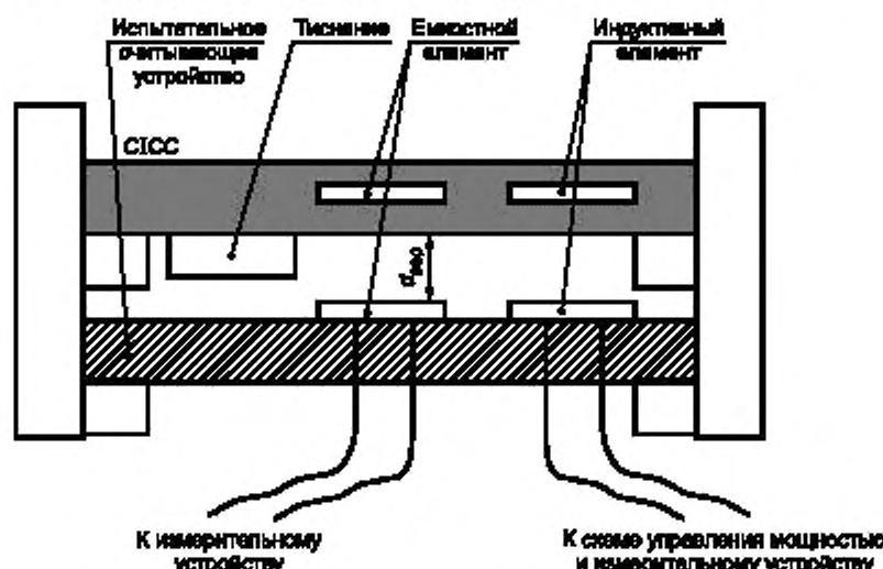
Рисунок Г.9 — Схема установки для испытаний СИСС
