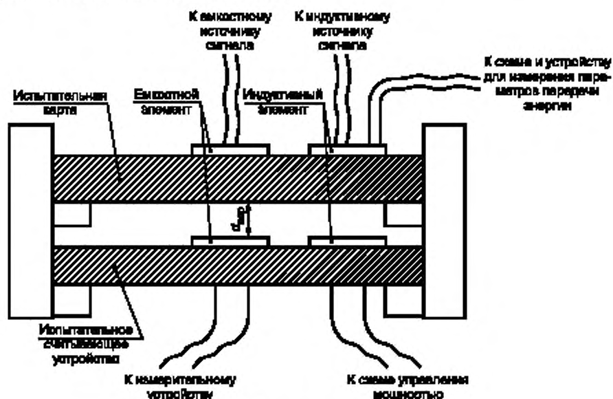
Рисунок Г.11 — Схема установки для калибровки
