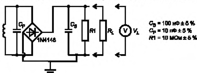
Рисунок А.1 — Схема для измерения магнитного поля
