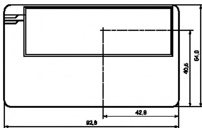
Рисунок Г.1 — Испытательная карта
