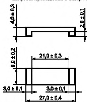
Рисунок Г.5 — Ферритовый сердечник и его размеры
