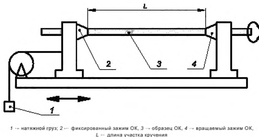
Рисунок 8 — Схема испытания ОК на воздействие осевого кручения
