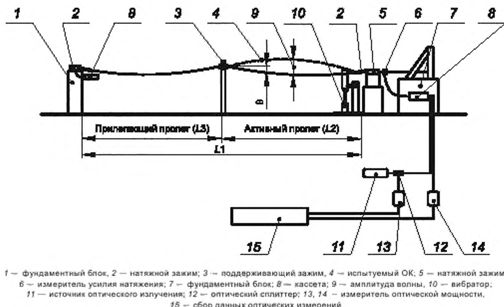
Рисунок 10 — Схема испытания ОК на воздействие галоирования
