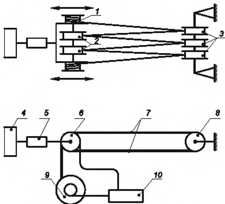
1 — барабаны крепления ОК; 2 — система натяжных роликов; 3 — система роликов-спутников; 4 — оборудование растяжения; 5 — датчик растягивающего усилия; 6 — система роликов и зажимы крепления ОК; 7 — участок ОК, подвергаемый растяжению; 8 — система роликов; 9 — ОК на барабане; 10 — средства измерений ОК
