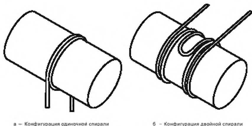
Рисунок 15 — Схема испытания ОК на воздействие статического изгиба
