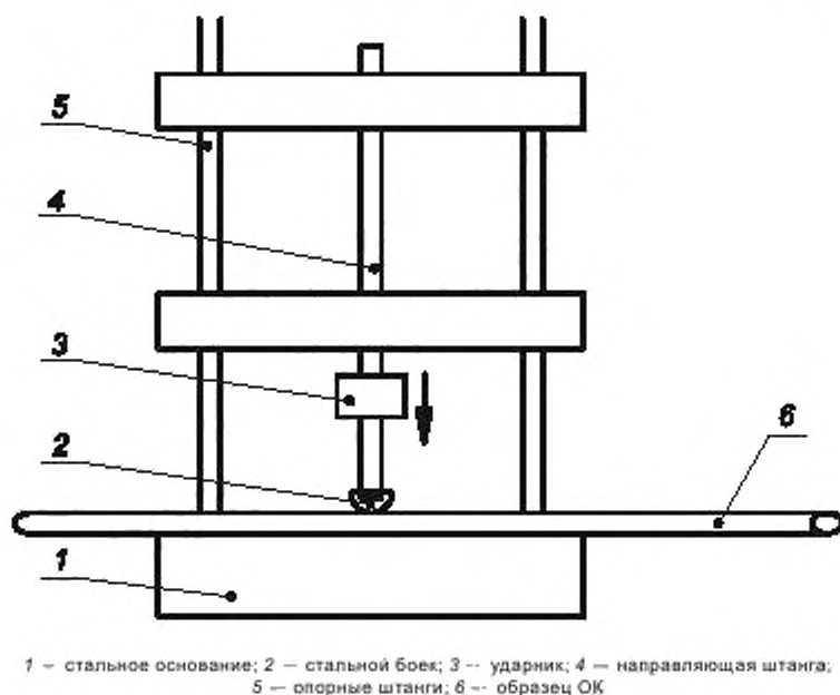
Рисунок 5 — Схема испытания ОК на воздействие удара
