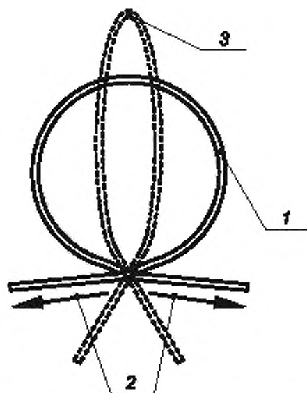
1 — петля ОМ, сформированная в начале испытания; 2 — направление приложения тягового усилия; 3 — конфигурация возникшего излома
