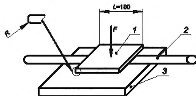
R , равный 5 мм, — радиус скругления кромок подвижной плиты; F — усилие, прикладываемое к подвижной плите в соответствии с документацией на ОК; L — длина плиты, l — перемещаемая плита, 2 — испытуемый образец ОК, 3 — неподвижная плита
