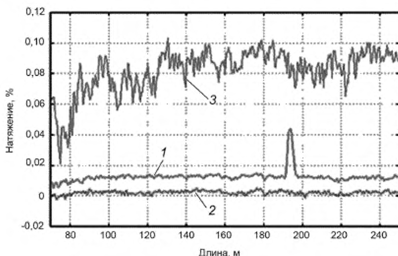
1 — ОВ имеет незначительное локальное натяжение; 2 — ОВ без натяжения; 3 — ОВ неоднородно натянуто по длине кабеля, деформация значительная
