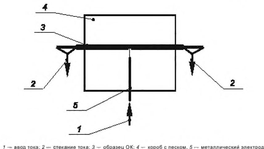
Рисунок 16 — Схема испытания ОК группы 3 на молниестойкость
