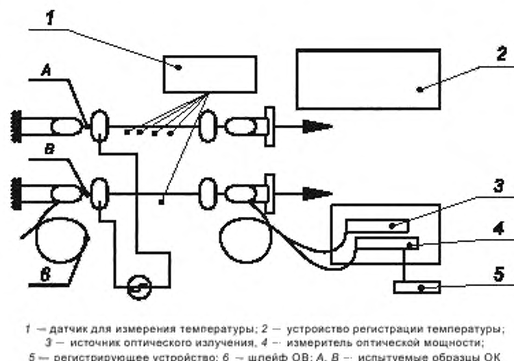
Рисунок 17 — Схема испытания ОК на протекание тока короткого замыкания ЛЭП
