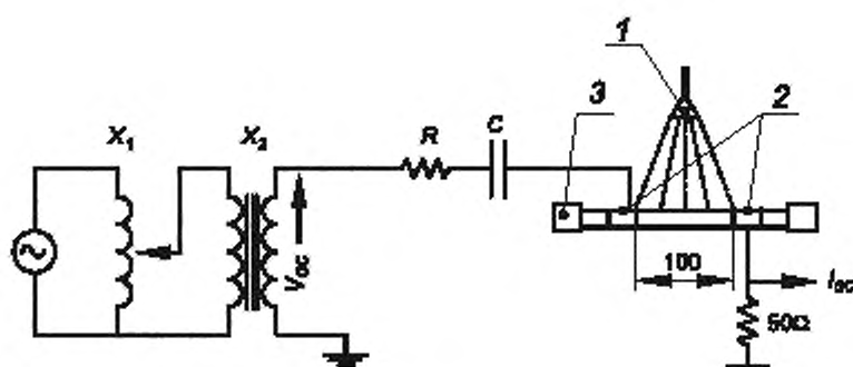
1 — распылитель солевого раствора; 2 — электроды из фольги; 3 — герметизированные концы ОК; X_1 — автотрансформатор; X_2 — высоковольтный трансформатор; V_{oc} — напряжение на высоковольтной обмотке; I_{sc} — ток при возникновении разряда; R , C — ограничители тока нагрузки
