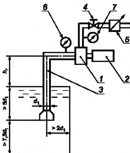
1 — насос, 2 — приводной двигатель; 3 — всасывающая линия, 4 — напорный вентиль, 5 — устройство для измерения подачи; 6, 7 — мановакуумметры
