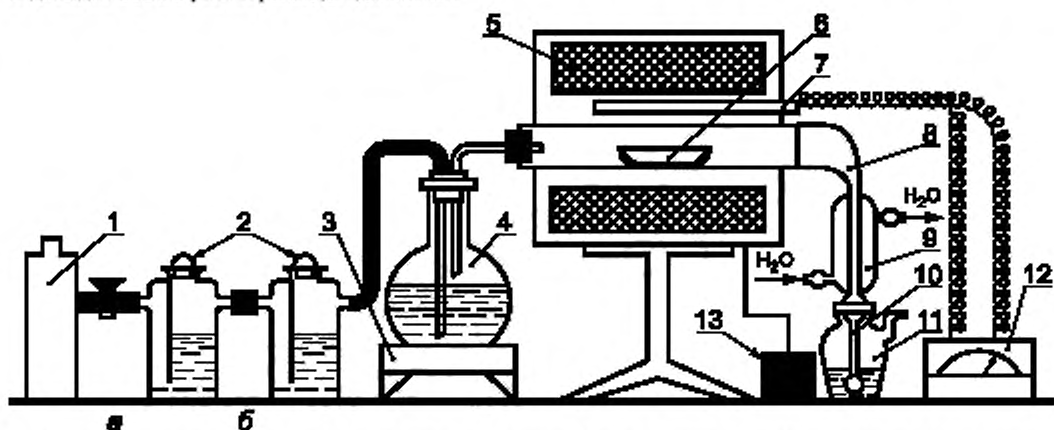
1 — баллон с газом; 2 — очистительные склянки; а — раствор \text{KMnO}_4 в растворе \text{NaOH} , б — дистиллированная вода; 3 — электролитка; 4 — парогенератор; 5 — трубчатая электронагревательная спираль; 6 — лодочка кварцевая; 7 — платина-платинородиевая термопара; 8 — кварцевая трубка; 9 — холодильник; 10 — отводная трубка; 11 — колба-приемник; 12 — милливольтметр; 13 — трансформатор напряжения для регулирования температуры печи
