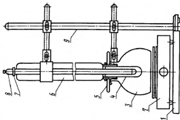
Схема плавыльника аппарата
