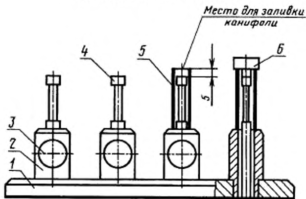
Схема станка для заливки продукта
