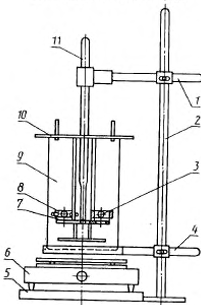
Схема основного блока аппарата
