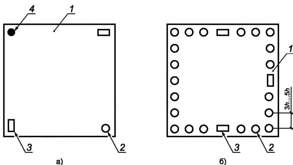
а) Опирание по четырем углам; б) Опирание по четырем сторонам
