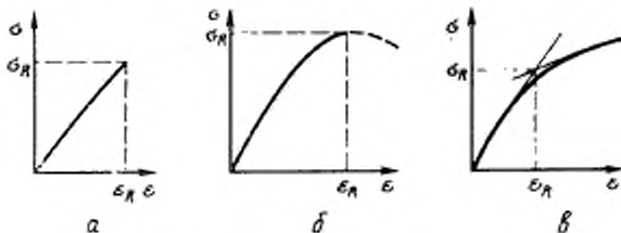
а—хрупкий тип деформирования; б—хрупко-пластический тип деформирования; в—пластический тип деформирования
