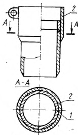
Режущее кольцо разрезное
