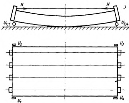
Схема расположения индикаторов при прогибе формы
