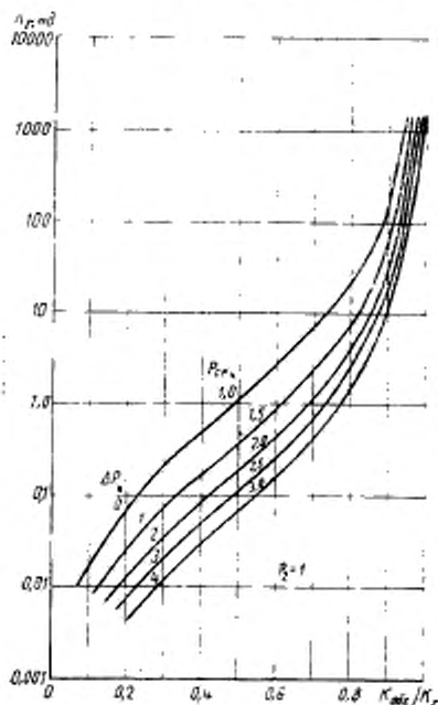
Номограмма для вычисления поправки к газопроницаемости за счет скольжения газа
