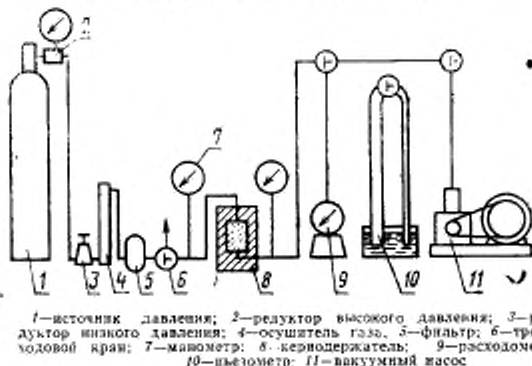
Принципиальная схема установки для определения газопроницаемости
