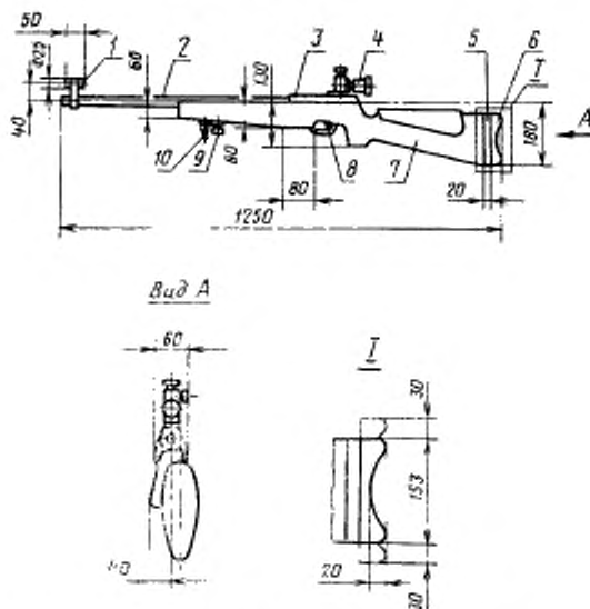
1 — основание мушкетера; 2 — ствол; 3 — коробка; 4 — прицел; 5 — прокладка; 6 — затылок приклада; 7 — ложа; 8 — спусковой крючок; 9 — упор для руки; 10 — антабля
