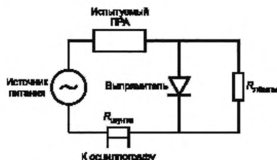
Рисунок 3 — Схема испытания пускового тока лампы
