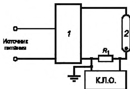
1 — испытуемый ПРА; 2 — номинальная лампа, К.Л.О. — осциллограф
