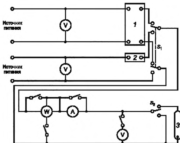
1 — испытуемый ПРА; 2 — ДОО; 3 — номинальная лампа
