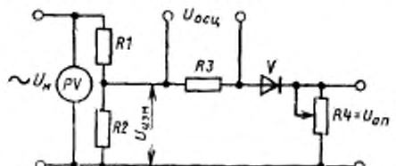
R1, R2, R3 — безындукционные резисторы. R4 — резистор; V — диод; U_n — номинальное напряжение; U_{изм} — измеряемое напряжение; U_{оп} — постоянное опорное напряжение; U_{осц} — амплитудное значение напряжения на входе осциллографа ( U_{осц} > U_{оп} ); PV — вольтметр
