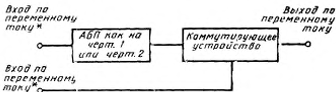
Единичный АБП с обводной цепью
