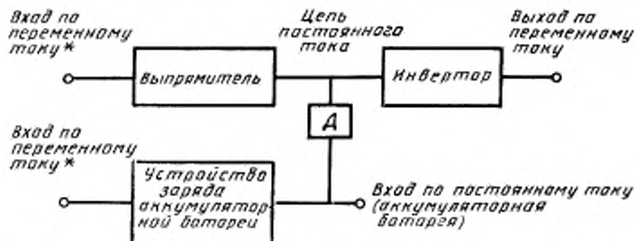
Единичный АБП с независимым зарядом аккумуляторной батареи
