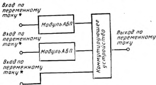
АБП с выделенным резервом с обводной цепью
