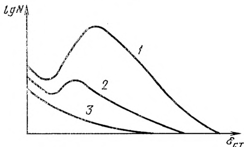
Зависимость усталостной выносливости от статической деформации для резин различного типа
