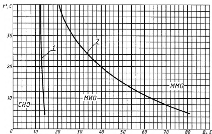
Зависимость условной вязкости от температуры
