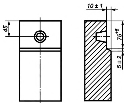
Рисунок А.10 — Размеры углублений для подвески. Вариант 5
