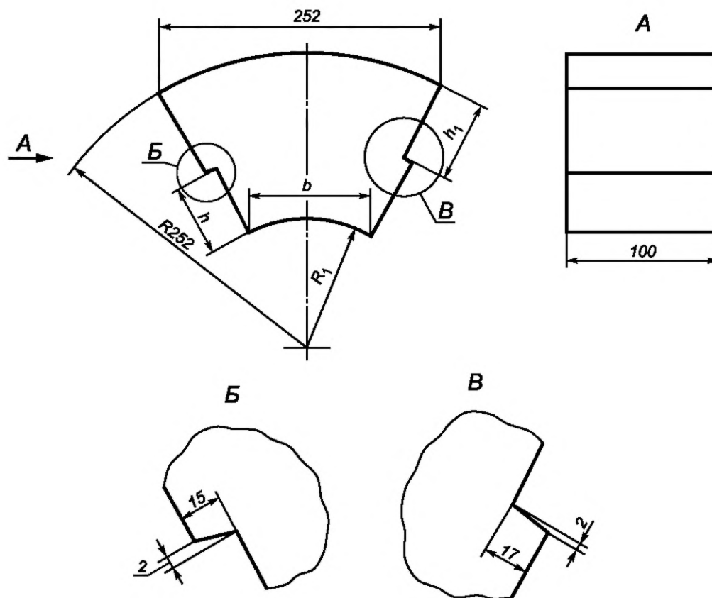
Рисунок 31 — Секторные фасонные изделия 144, 145
