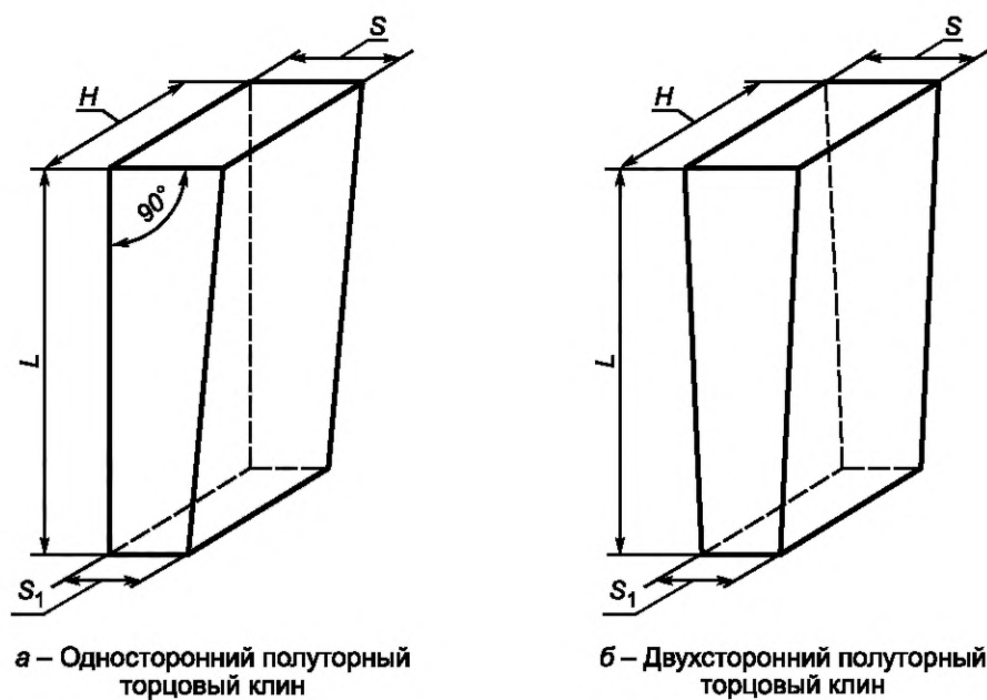
Рисунок 3 — Полуторные торцовые клины
