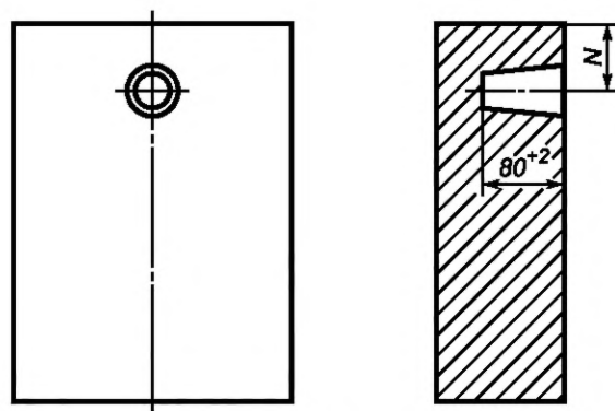
Рисунок А.4 — Размеры отверстий для штырей. Вариант 4
