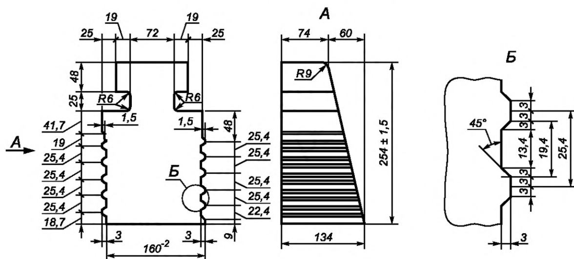
Рисунок 11 — Сводовое фасонное изделие 80
