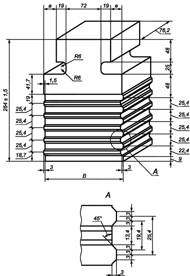
Рисунок 9 — Сводовые фасонные изделия 76—78
