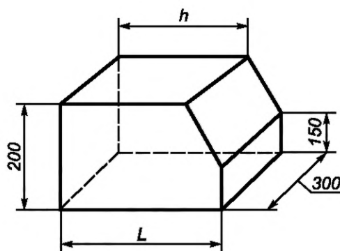
Рисунок 41 — Фасонные изделия 169, 170 (фасонный брусок)
