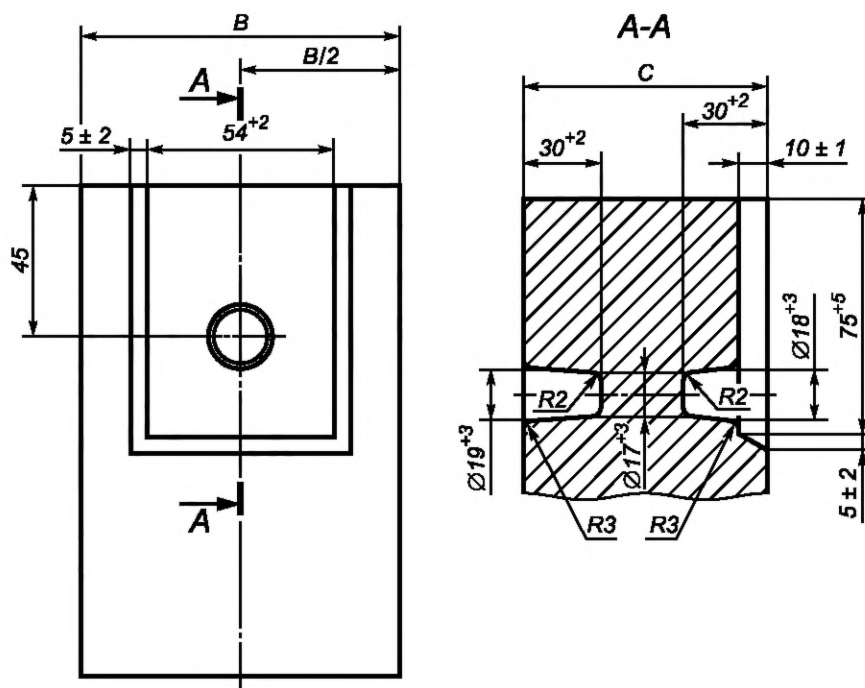
Рисунок А.7 — Размеры углублений для подвески. Вариант 2
