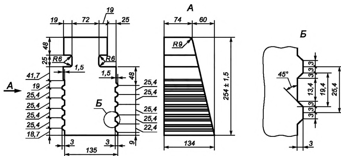
Рисунок 10 — Сводовое фасонное изделие 79
