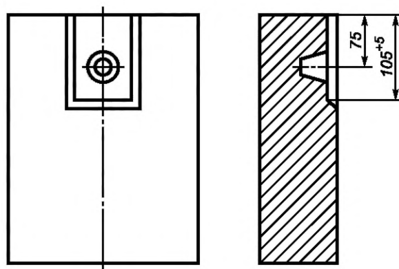
Рисунок А.8 — Размеры углублений для подвески. Вариант 3
