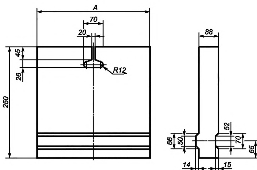
Рисунок 14 — Сводовые фасонные изделия 84, 85
