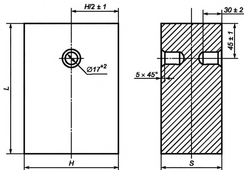
Рисунок А.1 — Размеры отверстий для штырей. Вариант 1
