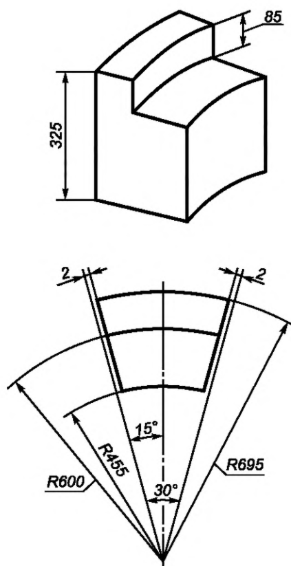
Рисунок 29 — Секторное фасонное изделие 142
