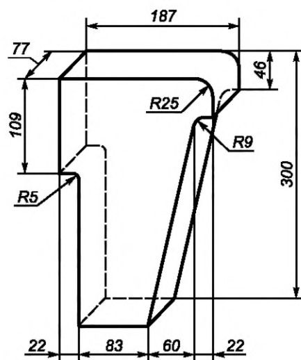
Рисунок 12 — Сводовое фасонное изделие 81
