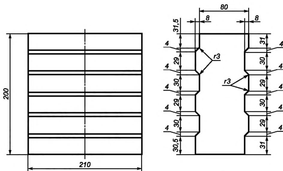
Рисунок 24 — Сводовое фасонное изделие 118
