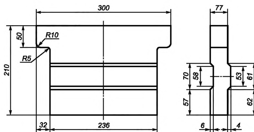
Рисунок 18 — Сводовое фасонное изделие 91
