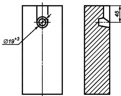
Рисунок А.9 — Размеры углублений для подвески. Вариант 4
