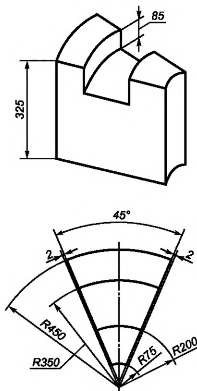
Рисунок 30 — Секторное фасонное изделие 143
