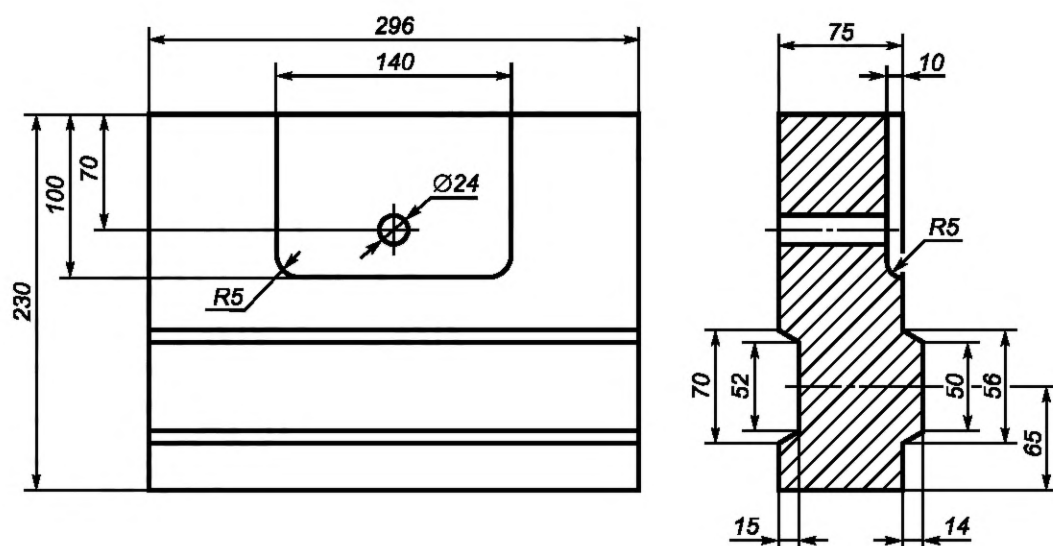
Рисунок 20 — Сводовое фасонное изделие 111
