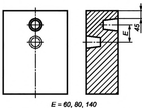
Рисунок А.3 — Размеры отверстий для штырей. Вариант 3
