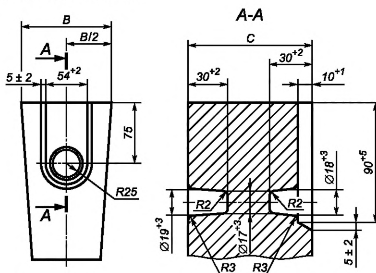
Рисунок А.6 — Размеры углублений для подвески. Вариант 1
