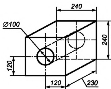
Рисунок 38 — Фасонное изделие с контрольным отверстием 166
