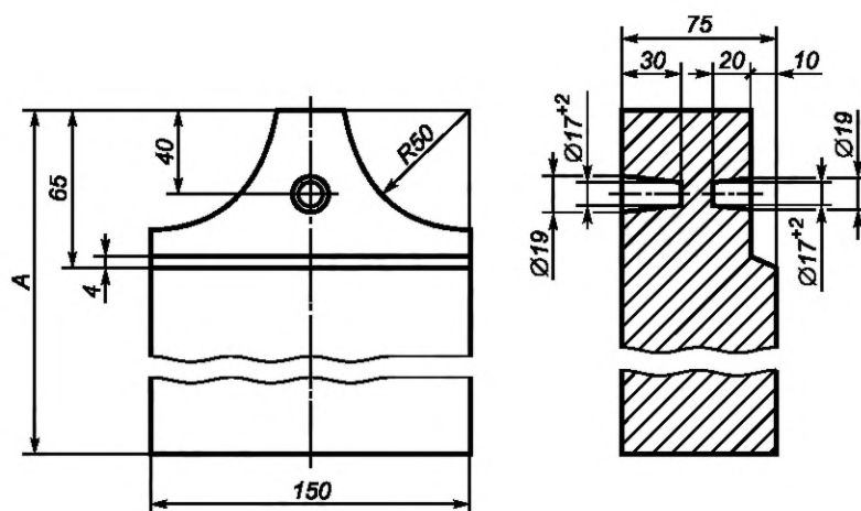
Рисунок 21 — Сводовые фасонные изделия 112, 113
