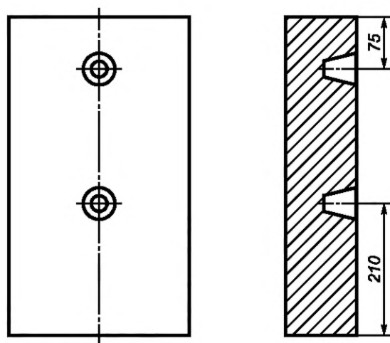
Рисунок А.5 — Размеры отверстий для штырей. Вариант 5
