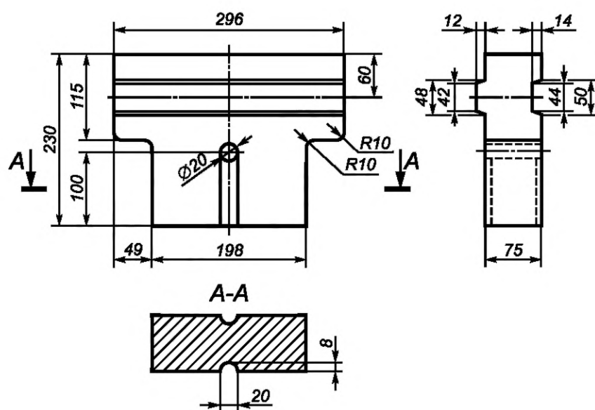
Рисунок 19 — Сводовое фасонное изделие 110
