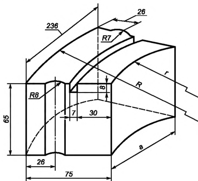
Рисунок 28 — Секторные фасонные изделия 103—109
