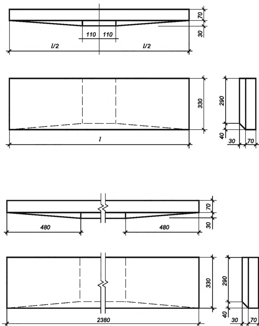
Рисунок 2 — Ступени типоразмеров ЛСС 12, ЛСС 15 и ЛСС 24
