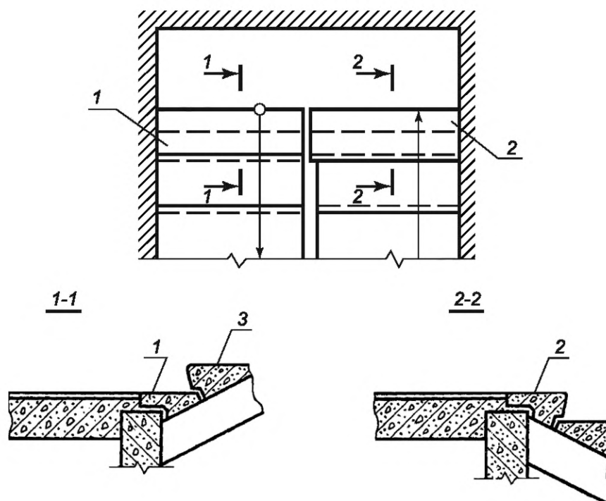
Рисунок А.1 — Междуетажные и этажные площадки
