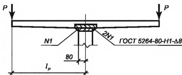
Рисунок 4 — Схема испытания ступеней типоразмеров ЛСС 12 и ЛСС 15
