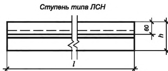
Рисунок 1 — Ступени типоразмеров ЛС, ЛСВ, ЛСП, ЛСН
