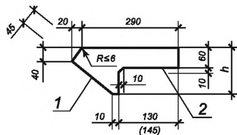
Рисунок 1 — Ступени типоразмеров ЛС, ЛСВ, ЛСП, ЛСН
